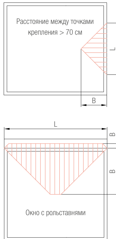
Рисунок 12: превышение максимально допустимого расстояния между точками крепления коробки
